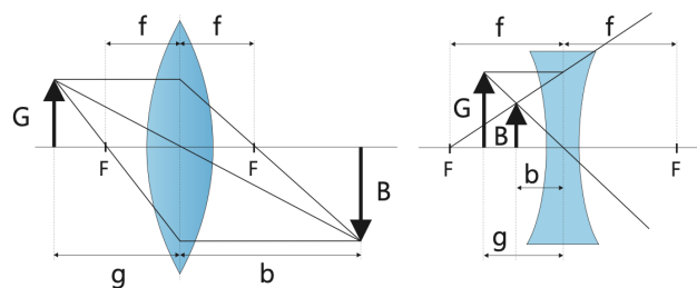
Abbildung 2.1: Strahlengang durch Linsen mit den charakteristischen Strahlen.
